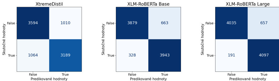
Obr. 2: Matice zámény pre binárne otázky
