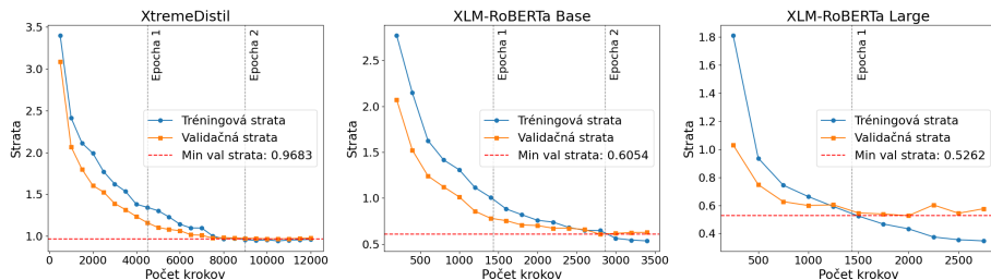
Obr. 1: Grafy loss funkcie
